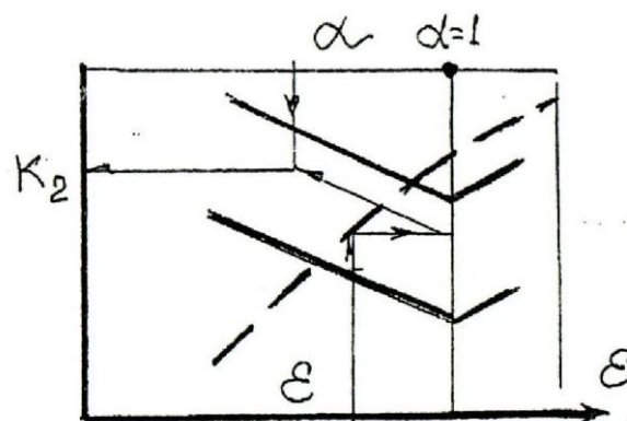
Рис. 2. Номограмма определения показателя адиабаты расширения K_2 для карбюраторного двигателя
