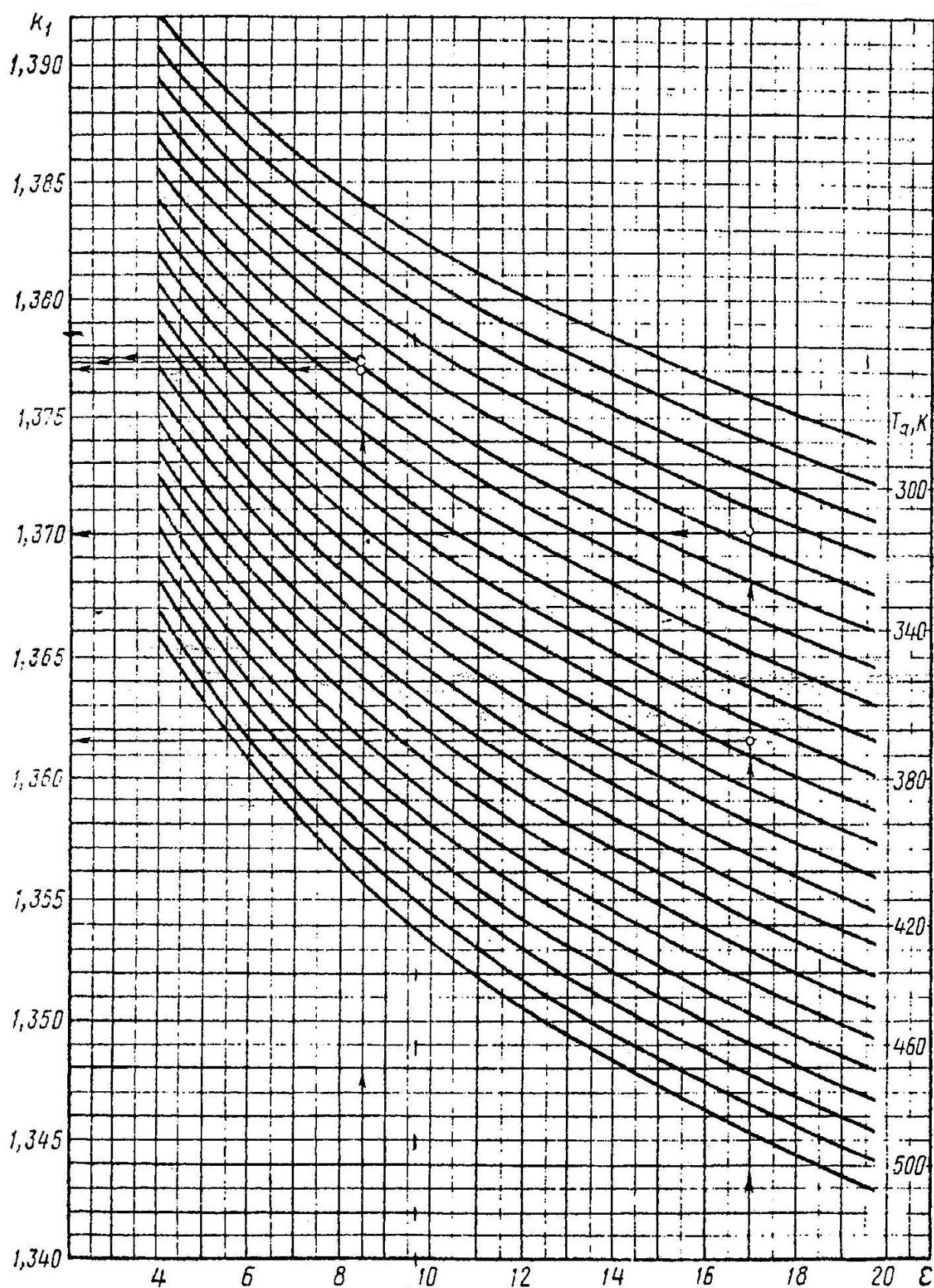
Рис. 1. Номограмма для определения показателя адиабаты сжатия K_1 . Пример: \varepsilon = 8,5 ; T_a = 340 K ; K_1 = 1,377 .
