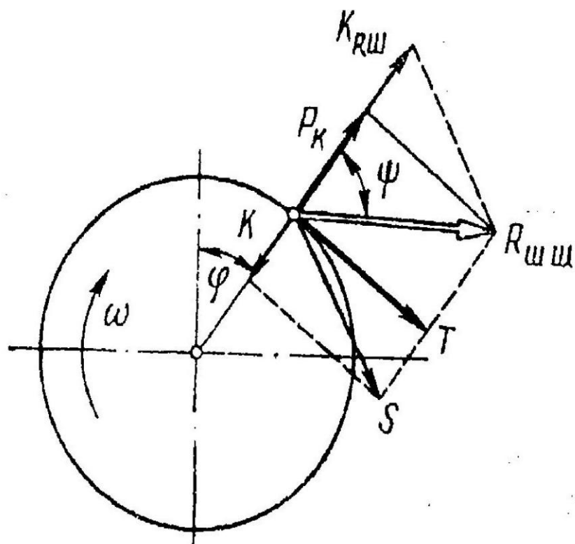
Рис. 10. Силы, действующие на шатунную шейку
