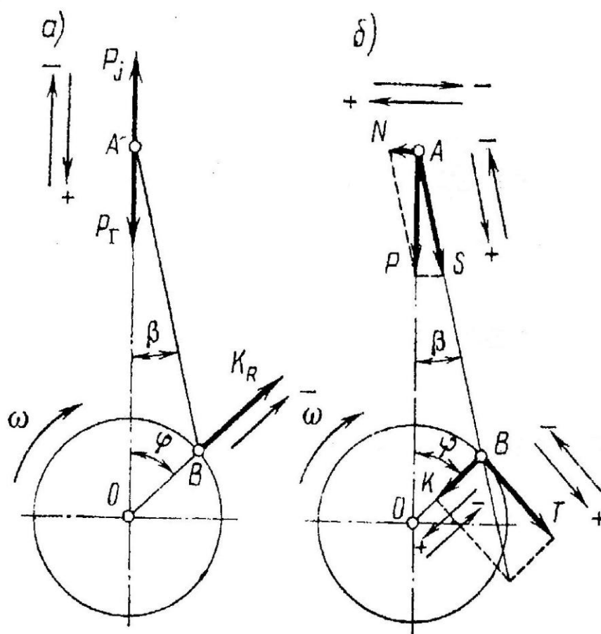
Рис. 9. Схема действия сил в КШМ: а – инерционных и газовых; б – суммарных
