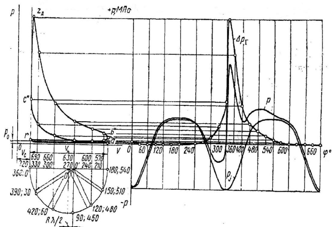
Рис. 7. Перестроение (развертка) индикаторной диаграммы в координатах P - \varphi
