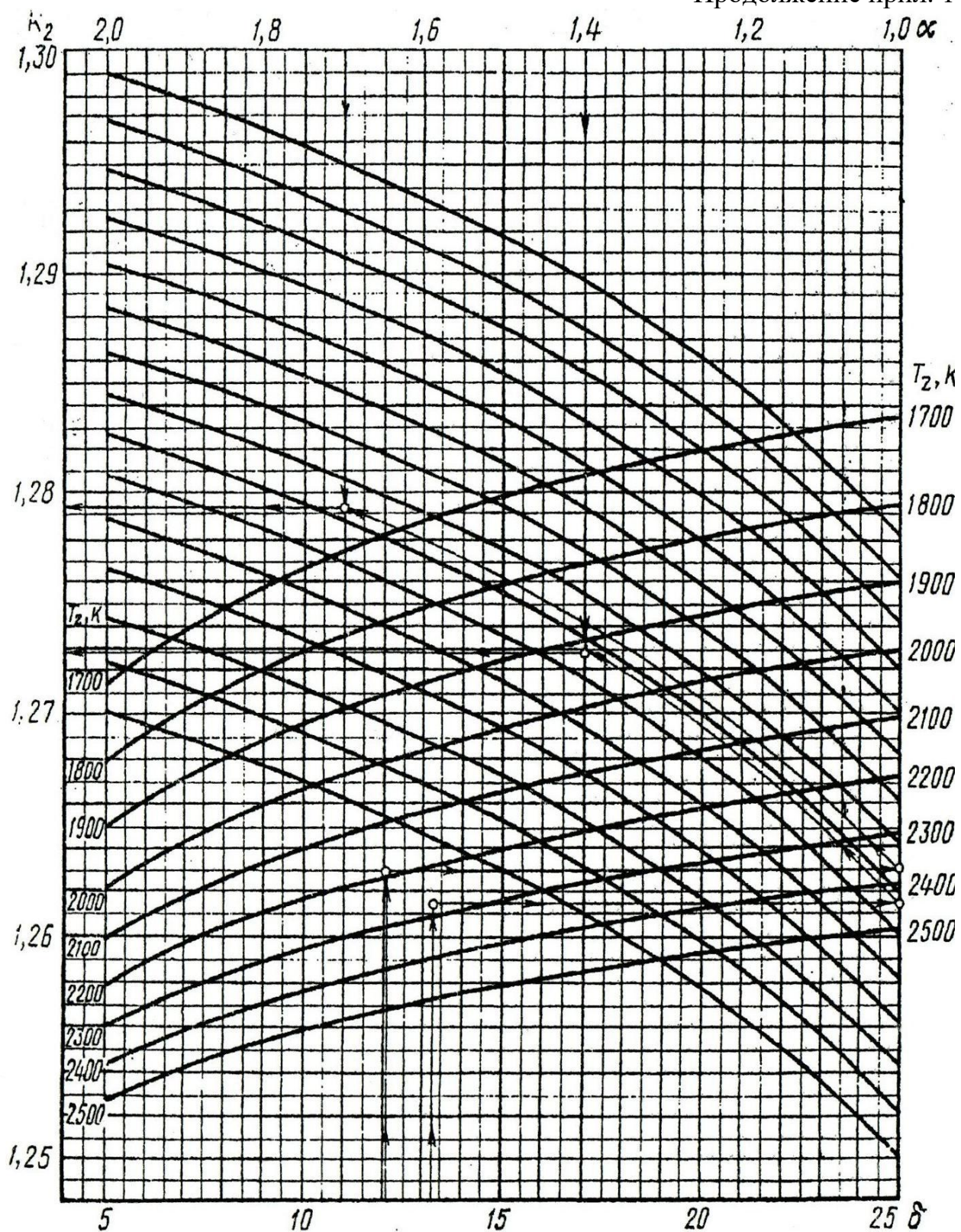
Рис. 3. Номограмма определения показателя адиабаты расширения K_2 для дизельного двигателя
