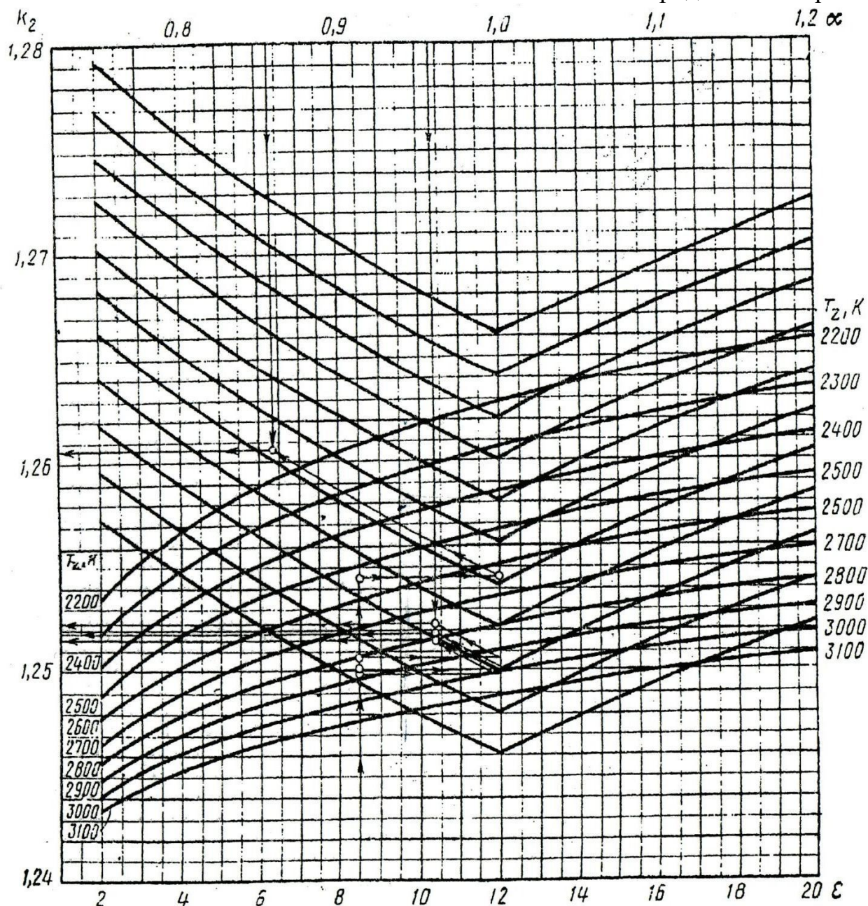
Рис. 2. Номограмма определения показателя адиабаты расширения K_2 для карбюраторного двигателя
