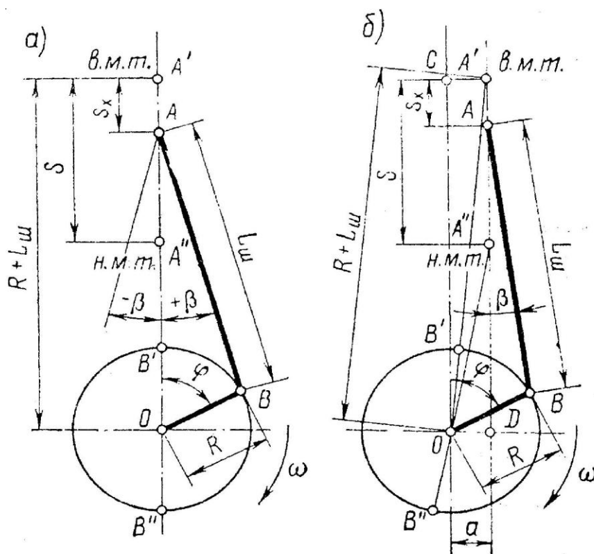
Рис. 3. Схемы кривошипно-шатунных механизмов: а – центрального; б – смещенного (дезаксиального)
