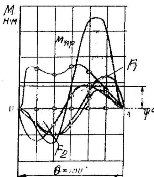
Рис. 12. График суммарного момента 4 – цилиндрового двигателя при равномерном чередовании рабочих процессов:
