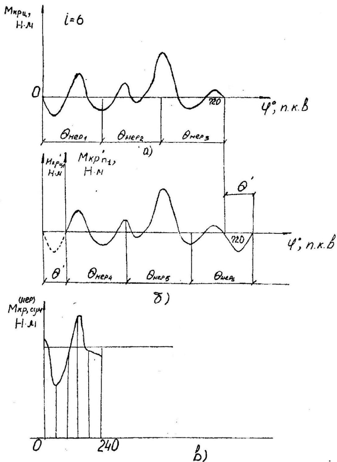
Рис. 13. Построение графика M_{KPi, \text{сум}} при неравномерном чередовании рабочих процессов: а – исходный график M_{KPi} ; б – преобразованный график M_{KPi} ; в – график суммарного момента M_{KPi, \text{сум}}
