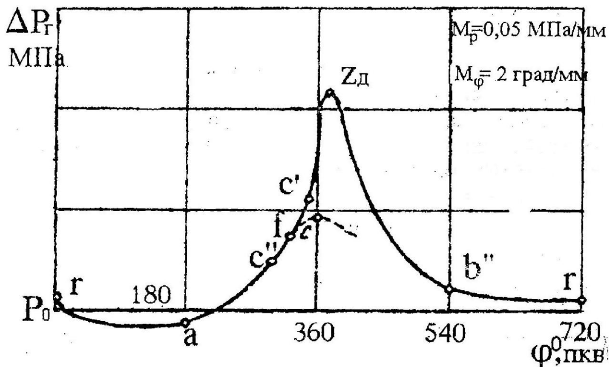
Рис. 8. Диаграмма удельных сил давления газов карбюраторного двигателя
