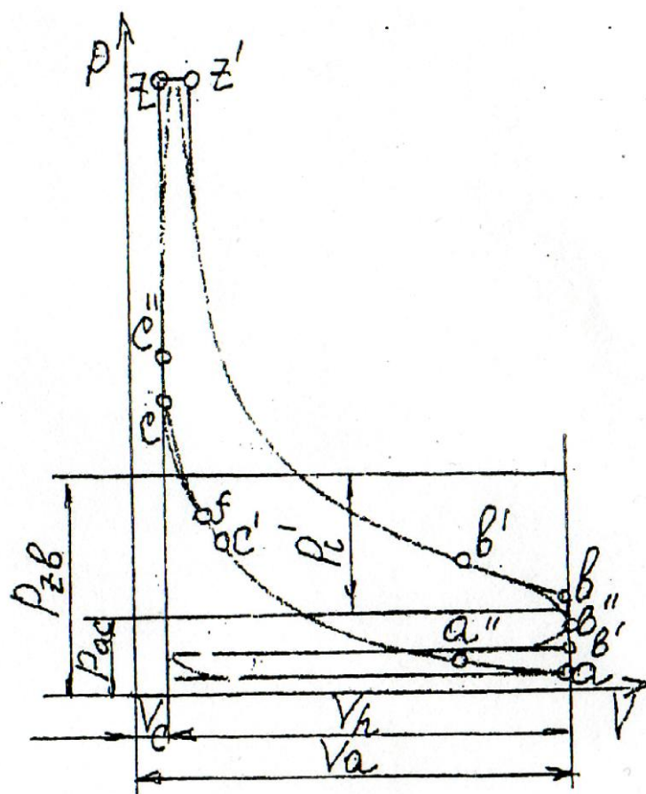
Рис. 2. Индикаторная диаграмма дизеля
