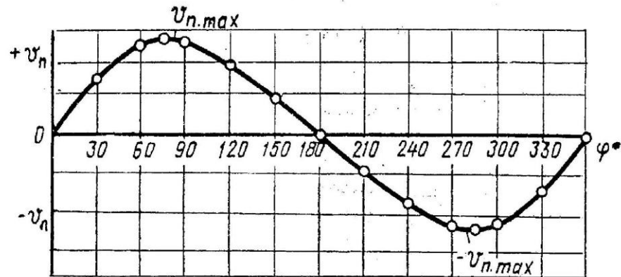
Рис. 5. Построение кривых скорости поршня аналитическим методом
