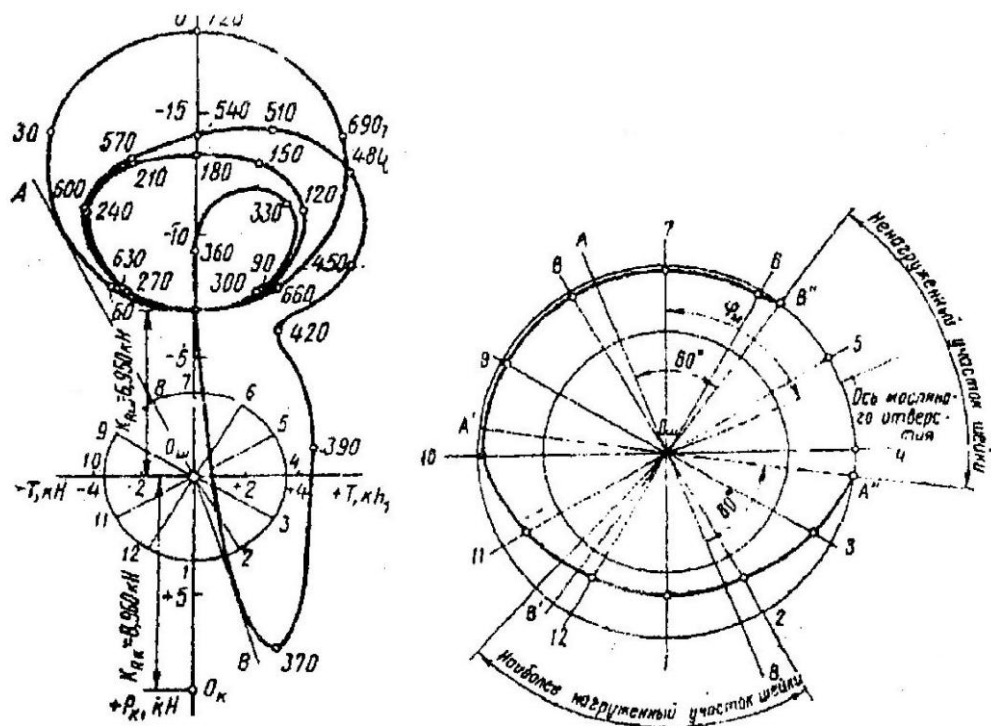
Рис. 15. Полярная диаграмма и диаграмма износа шатунной шейки
