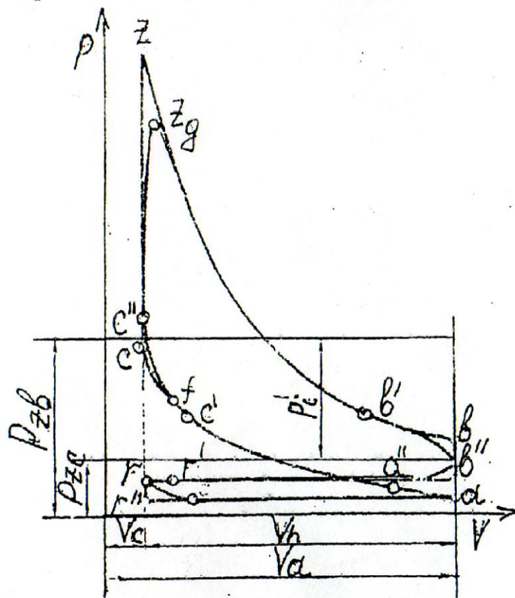
Рис. 1. Индикаторная диаграмма карбюраторного двигателя
