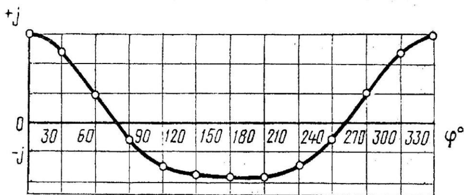
Рис. 6. Построение кривых ускорения поршня аналитическим методом
