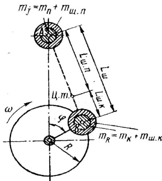
Рис. 11. Приведение масс деталей КШМ
