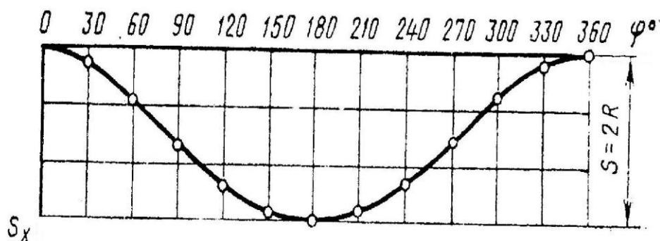
Рис. 4. Построение кривых перемещения поршня аналитическим методом
