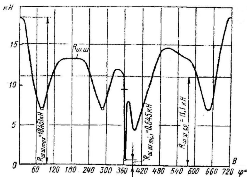
Рис. 14. Диаграмма результирующей силы R_{шш} в прямоугольных координатах
