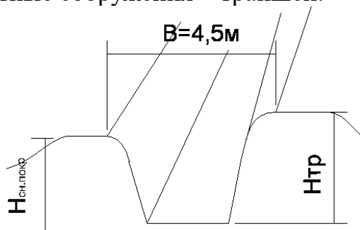
Рис. 4. Схема траншеи
