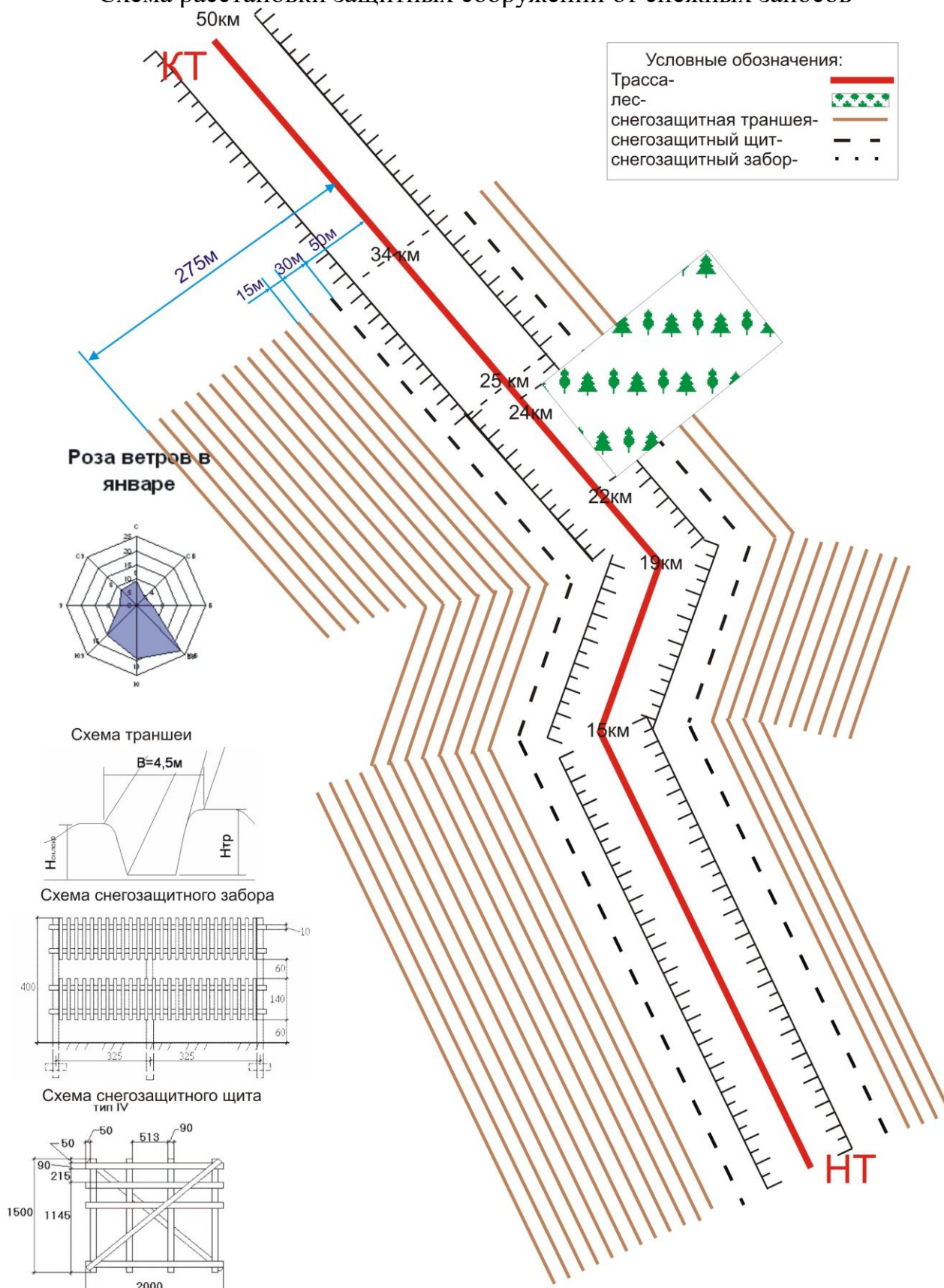
Схема расстановки защитных сооружений от снежных заносов
