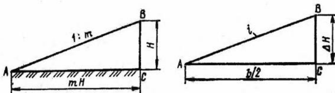
Рис.13. Схема к определению крутизны откоса насыпи и поперечного уклона проезжей части
