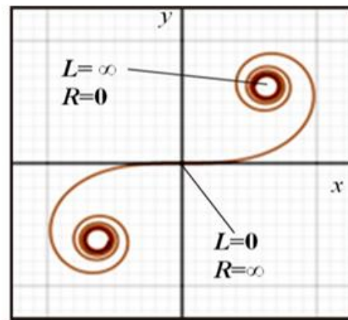
Рис.7. График клотоиды
