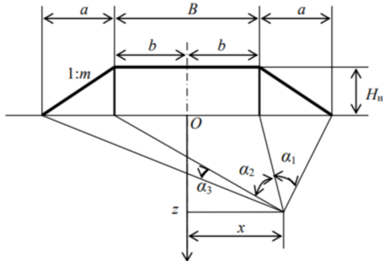
Рис.2. Расчётная схема для оценки осадки насыпи
