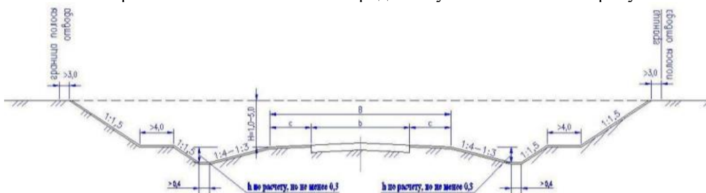
Рис. 6. Выемка с закуветными полками
