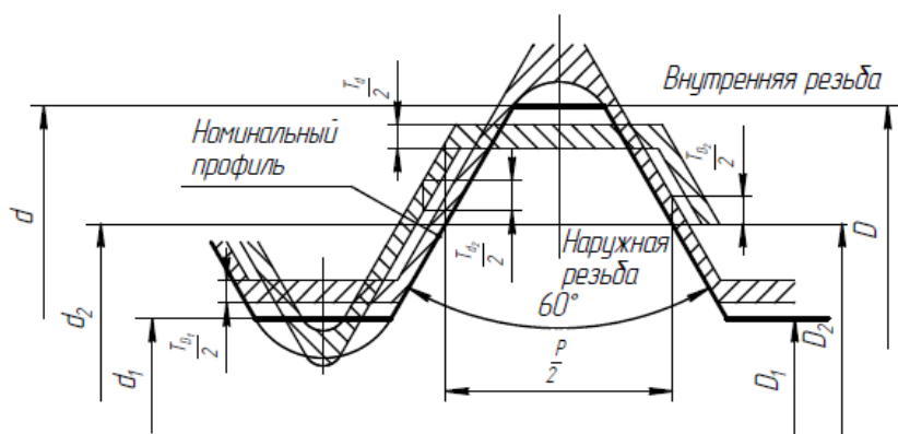
Рисунок 3.4 Расположение полей допусков метрической резьбы болта и гайки с натягом
