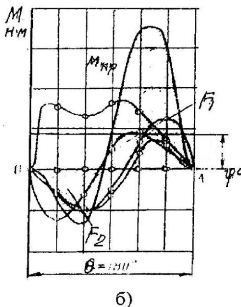
Рис. 12. График суммарного момента 4 – цилиндрового двигателя при равномерном чередовании рабочих процессов:
