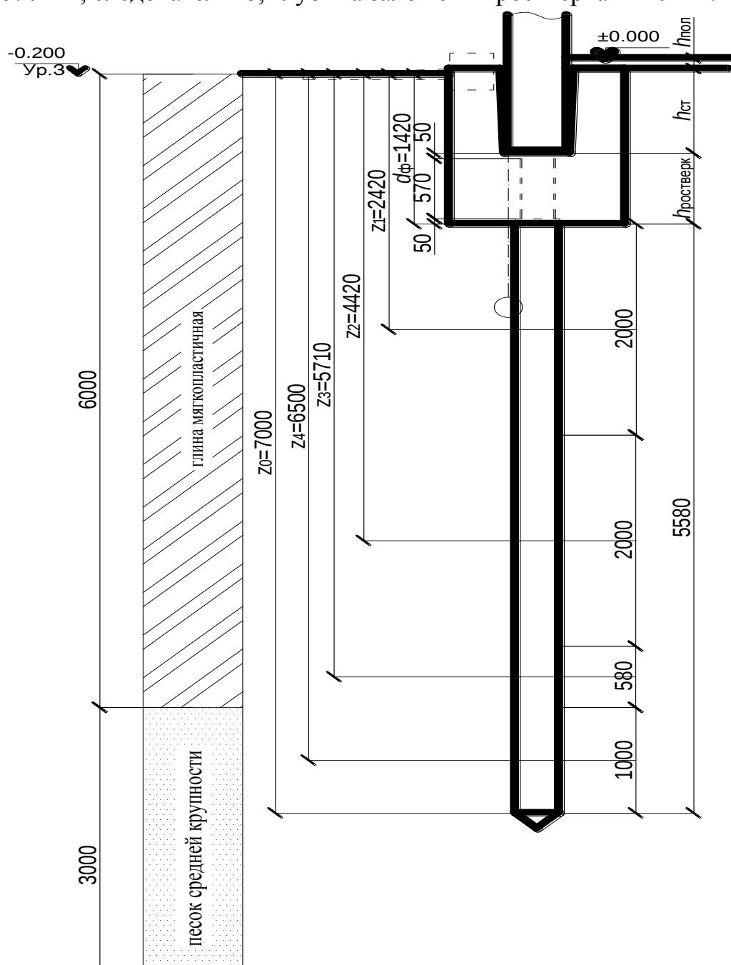
Рис. 7. Назначение конструктивной глубины заложения ростверка и длины свай
