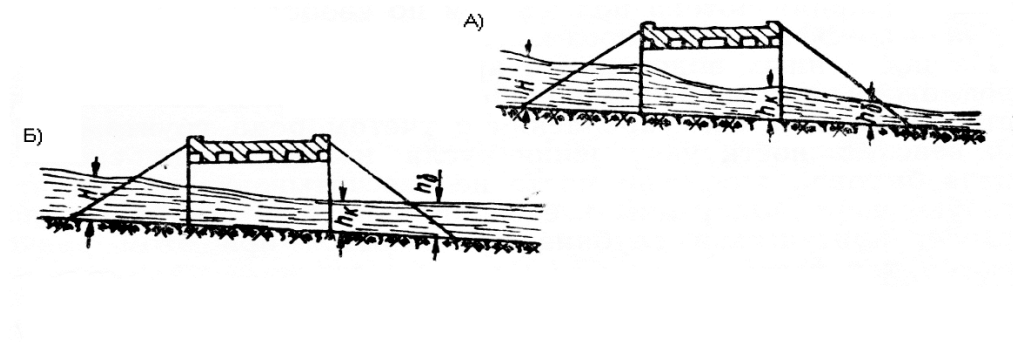
Рис. 17. Протекание воды под малым мостом: а- свободное истечение; б- несвободное истечение
