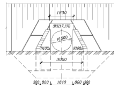
Разрез 1-1 насыпь по показанию
