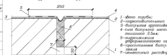
Узел А. М1:2,5 Гидроизоляция трубы
